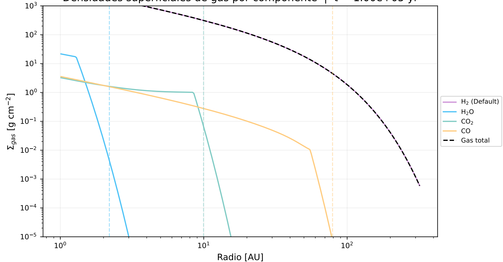
Densidades superficiales de gas por componente | t = 1.00\text{e}+05 yr
